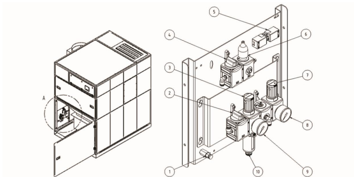
Fig. 12: Unità pneumatica
